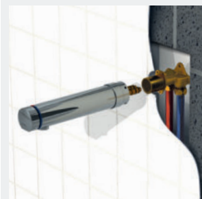
Niche béton
