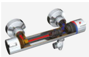
Doorsnede H9768BEL: kleine hoeveelheid water, thermische isolatie Ref. DELABIE: Coupe3D_H9768BEL + 880
