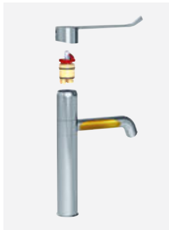
Mechanische wastafelmengkraan met draaibare uitloop Ref. DELABIE: 2564T1BEL
