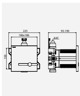
TEMPOMATIC dubbele bediening op batterijen DELABIE ref.: 464PBOX-464006
