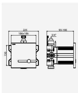
TEMPOMATIC dubbele bediening op netspanning DELABIE ref.: 464SBOX-464000
