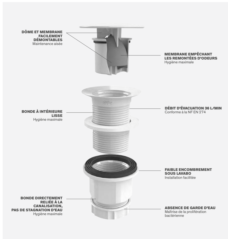
Coupe 621W : bonde sans eau Réf. DELABIE : Coupe3D_621W
