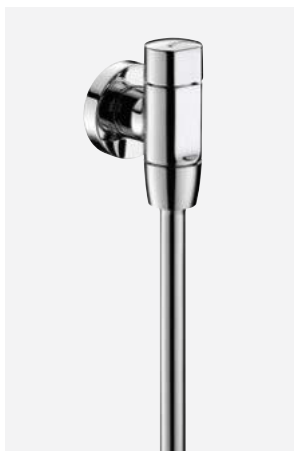
Robinet d'urinoir temporisé TEMPOFLUX Réf. DELABIE : 778755
