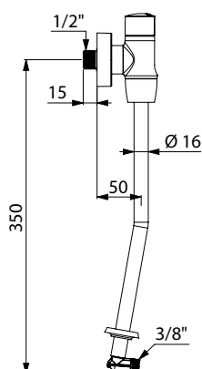
Robinets d'urinoir temporisés TEMPOFLUX Réf. DELABIE : 778759, 778757, 778755
